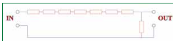
Fig.4: Viene qui posto in evidenza che, adottando la tecnica di regolazione del livello più semplice, i componenti passivi che il segnale è costretto ad attraversare, soprattutto per le posizioni relative ai livelli più bassi, sono assai numerosi. Inutile dire che per il suo preamplificatore top il costruttore Ayon non ha scelto questa soluzione, ma l'altra prospettata in Fig.3/b, ben più performante, benché di più complessa ed onerosa realizzazione.
